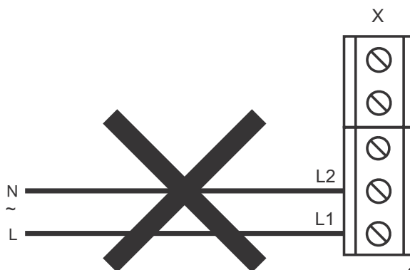
Wiring diagram 15
